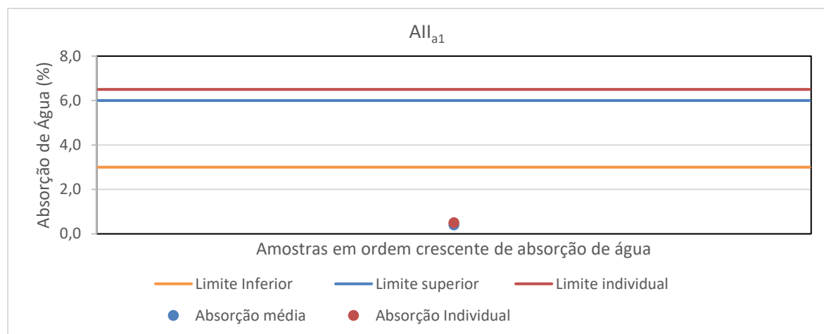
Figura 11: Valores médio e individual máximo de absorção de água para o produto do grupo de absorção de água AI_{a1} .
