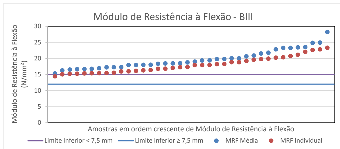
Figura 33: Valores médio e individual mínimo do módulo de resistência à flexão dos produtos do grupo de absorção de água BIII.
