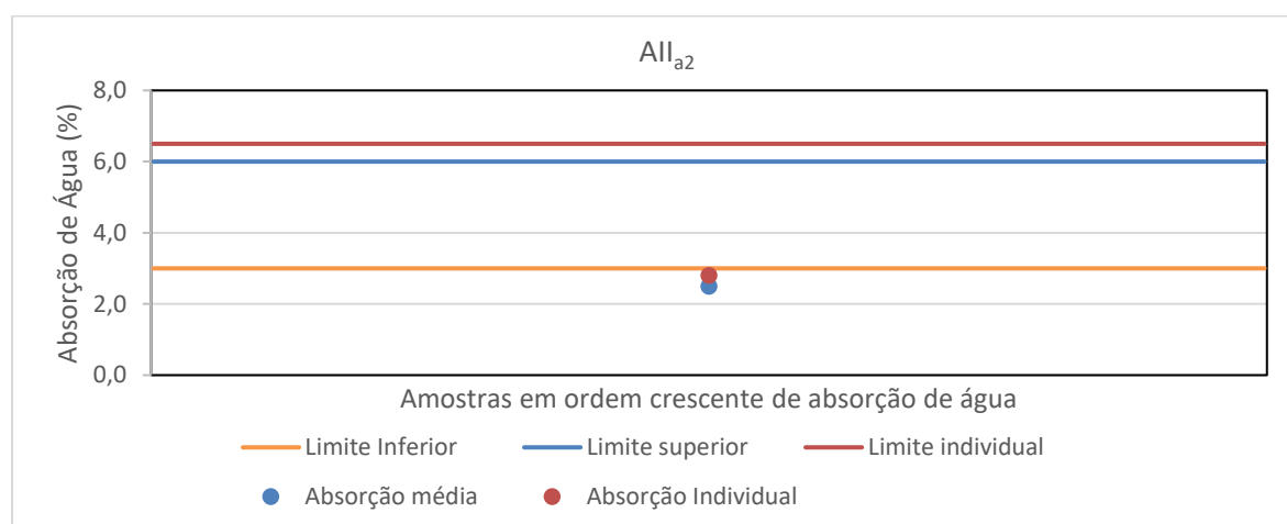
Figura 12: Valores médio e individual máximo de absorção de água para o produto do grupo de absorção de água AI_{a2} .
