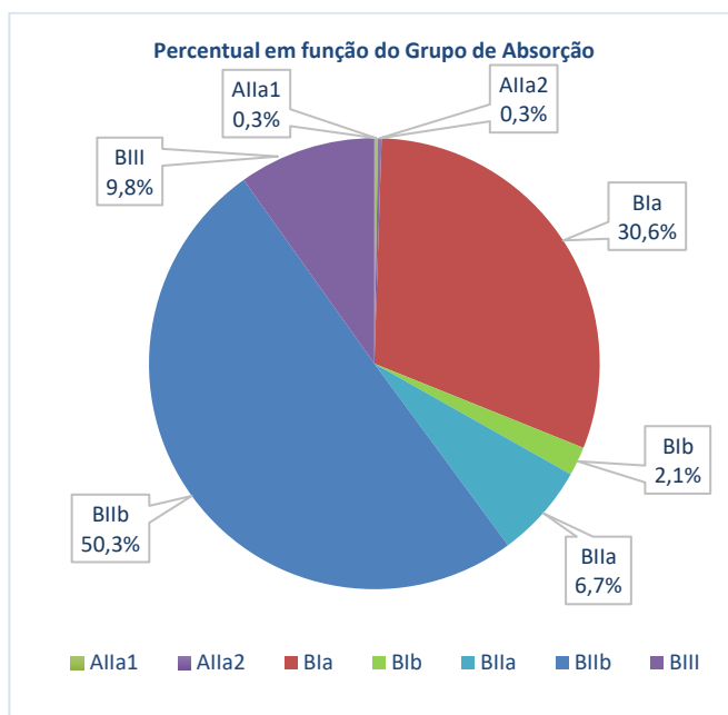
Figura 4: Distribuição dos produtos avaliados em função do grupo de absorção de água.
