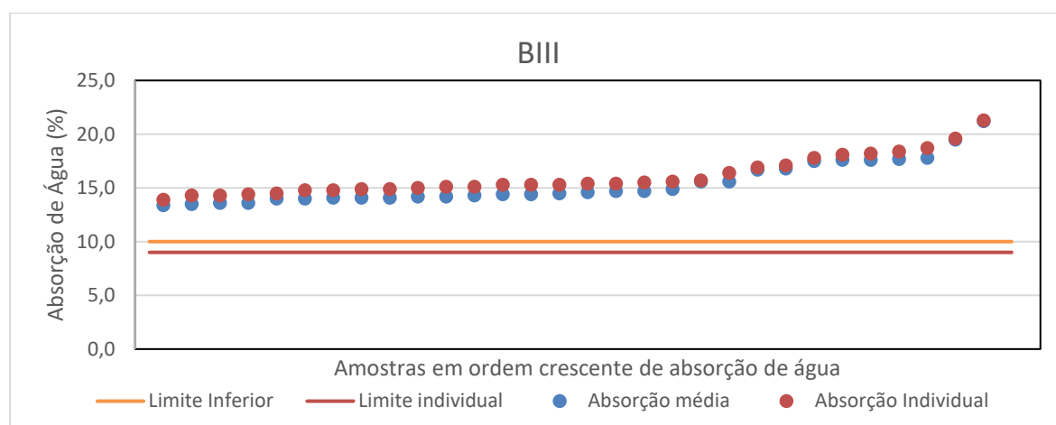
Figura 17: Valores médio e individual mínimo de absorção de água para os produtos do grupo de absorção de água BIII.
