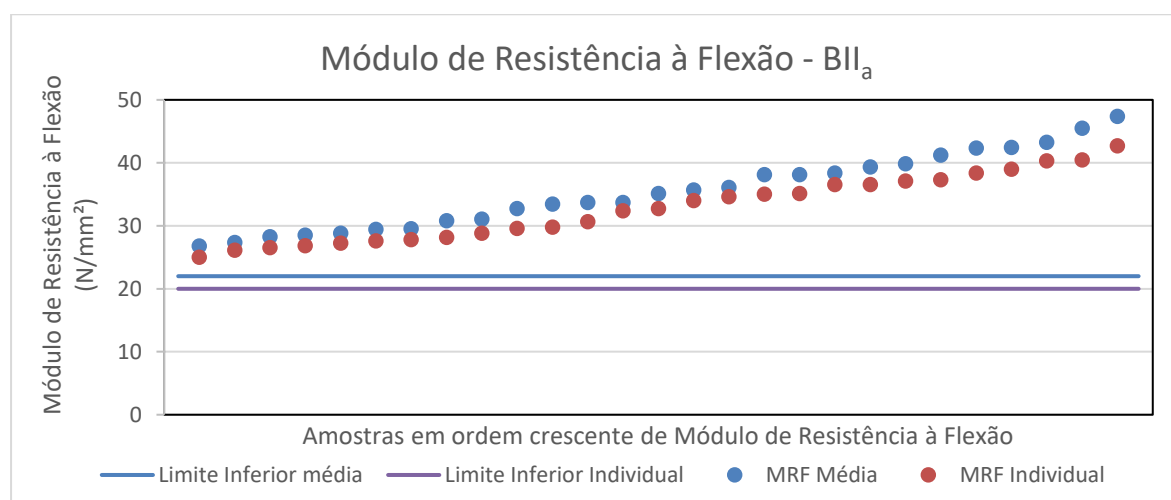
Figura 31: Valores médio e individual mínimo do módulo de resistência à flexão dos produtos do grupo de absorção de água BIIa.
