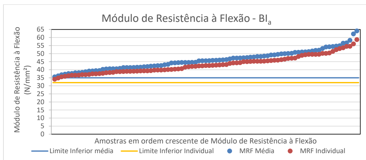
Figura 29: Valores médio e individual mínimo do módulo de resistência à flexão dos produtos do grupo de absorção de água Bl a .
