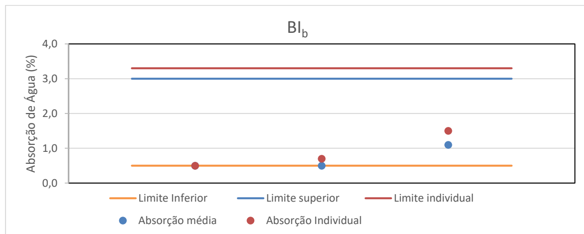
Figura 14: Valores médio e individual máximo de absorção de água para os produtos do grupo de absorção de água BIb.
