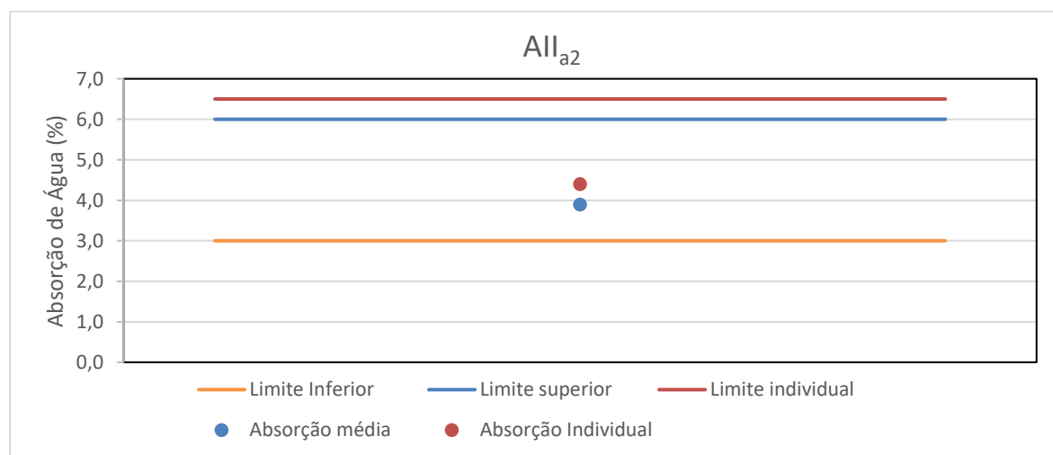
Figura 12: Valores médio e individual máximo de absorção de água para o produto do grupo de absorção de água AII a2 .
