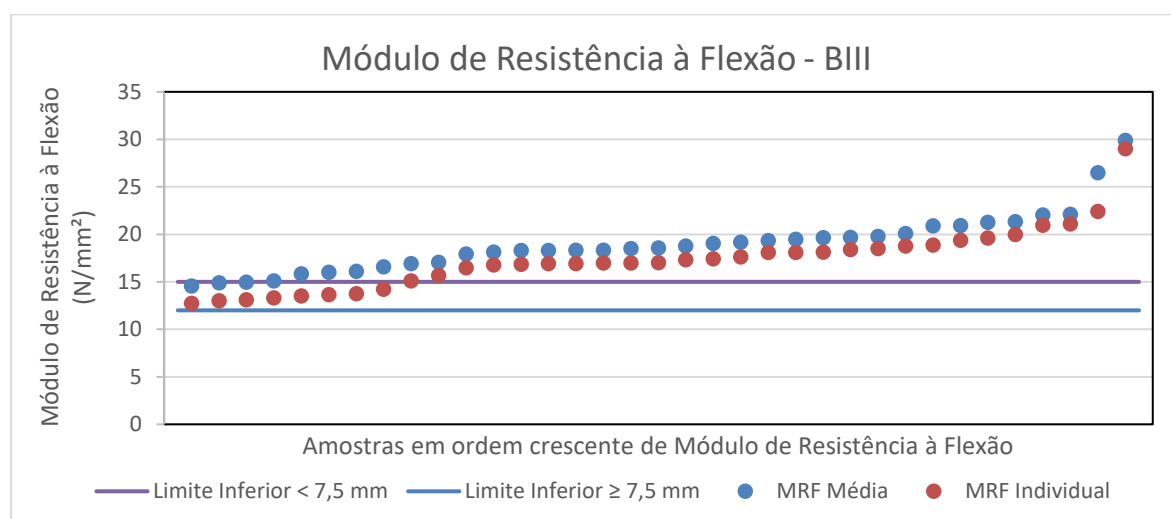
Figura 33: Valores médio e individual mínimo do módulo de resistência à flexão dos produtos do grupo de absorção de água BIII.
