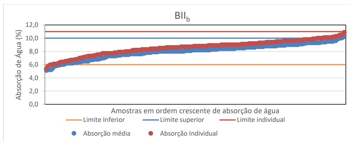
Figura 16: Valores médio e individual máximo de absorção de água para os produtos do grupo de absorção de água BIIb.
