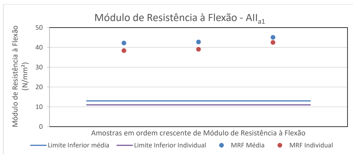
Figura 27: Valores médio e individual mínimo do módulo de resistência à flexão dos produtos do grupo de absorção de água All a1 .
