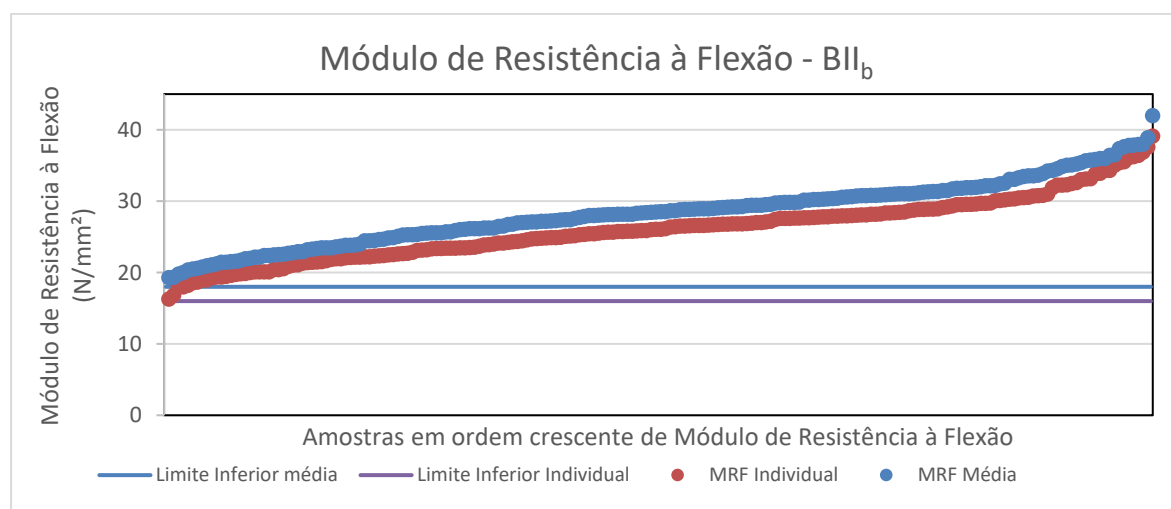
Figura 32: Valores médio e individual mínimo do módulo de resistência à flexão dos produtos do grupo de absorção de água BIIb.
