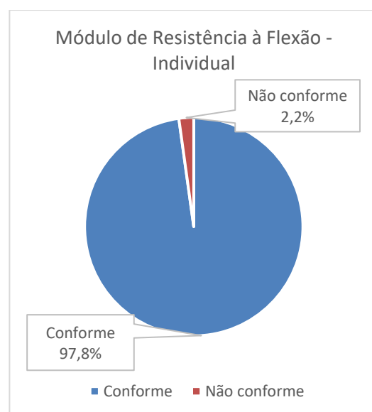
(b) Conformidade do valor individual de módulo de resistência a flexão em função dos grupos de absorção de água
