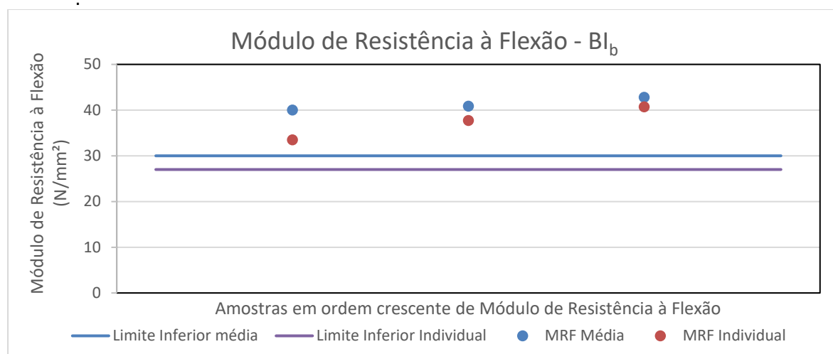
Figura 30: Valores médio e individual mínimo do módulo de resistência à flexão dos produtos do grupo de absorção de água Bl b .
