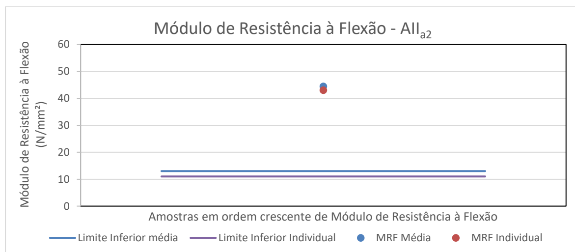
Figura 28: Valores médio e individual mínimo do módulo de resistência à flexão dos produtos do grupo de absorção de água All a2 .
