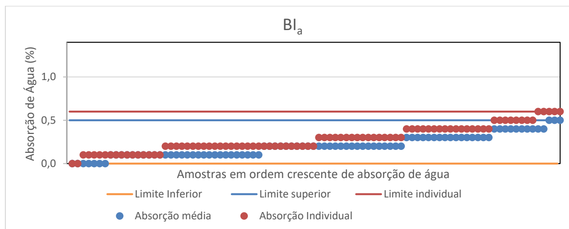
Figura 13: Valores médio e individual máximo de absorção de água para o produto do grupo de absorção de água BIa.
