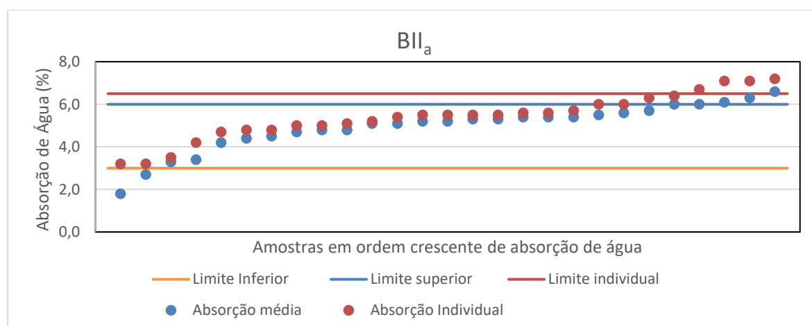
Figura 15: Valores médio e individual máximo de absorção de água para os produtos do grupo de absorção de água BIIa.
