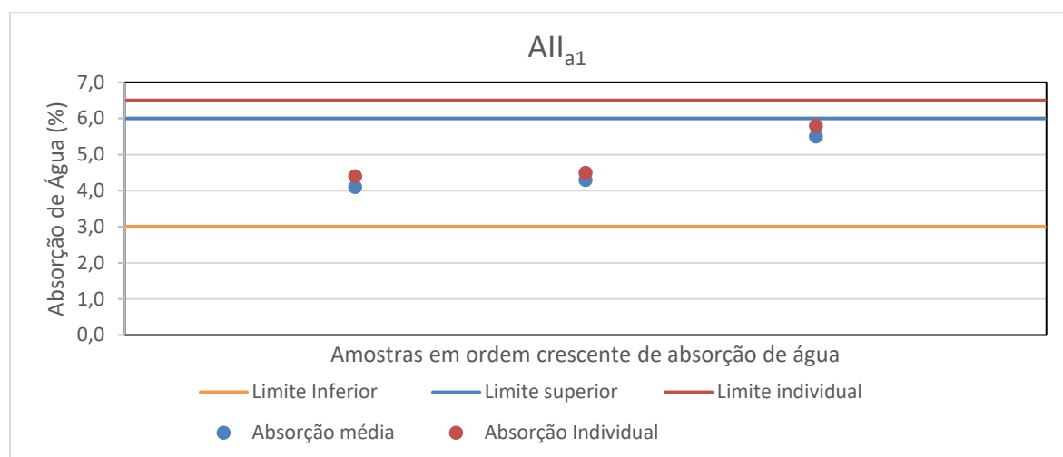
Figura 11: Valores médio e individual máximo de absorção de água para o produto do grupo de absorção de água AII a1 .
