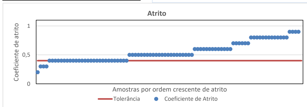
Figura 47: Resultados de determinação do coeficiente de atrito dos produtos avaliados.
