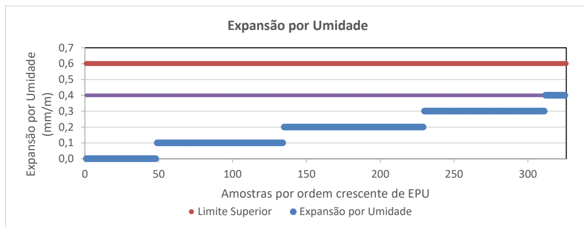
Figura 39: Resultados da determinação da expansão por umidade dos produtos.
