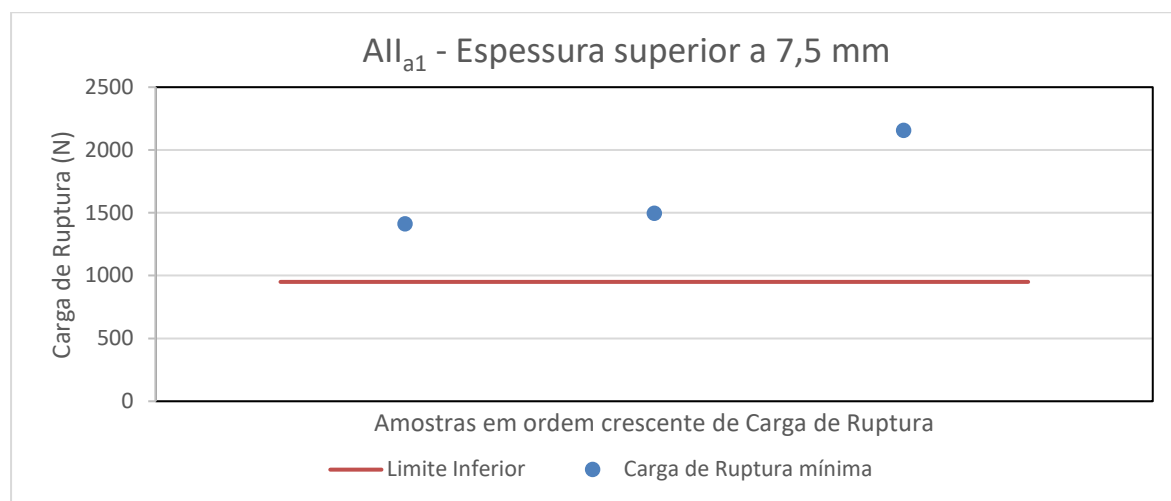
Figura 19: Valor mínimo de carga de ruptura dos produtos avaliados do grupo de absorção de água AI_{a1} .
