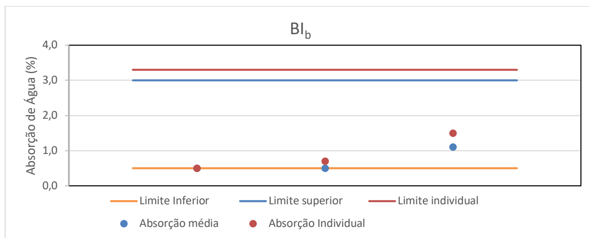
Figura 14: Valores médio e individual máximo de absorção de água para os produtos do grupo de absorção de água Bl b .
