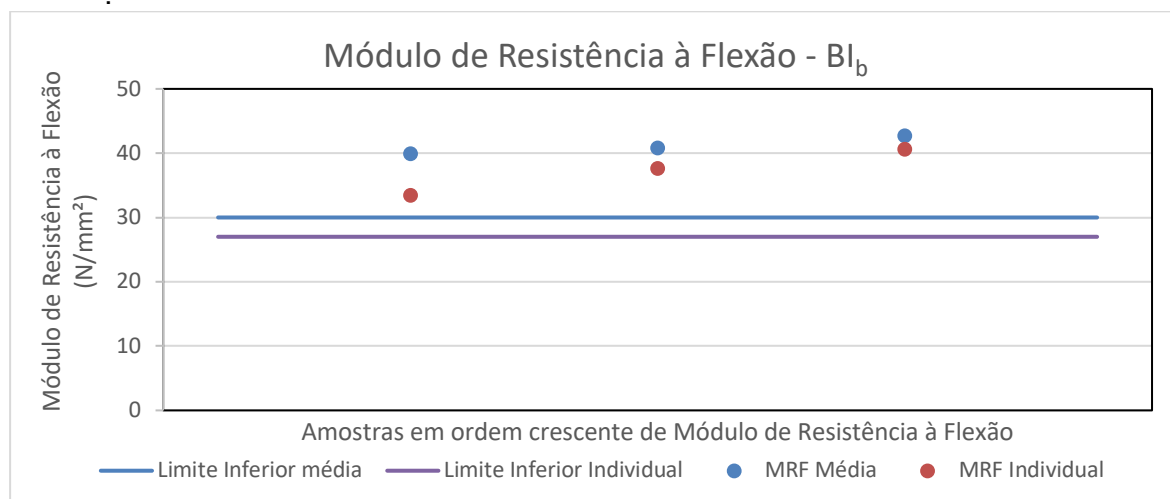
Figura 30: Valores médio e individual mínimo do módulo de resistência à flexão dos produtos do grupo de absorção de água BIb.
