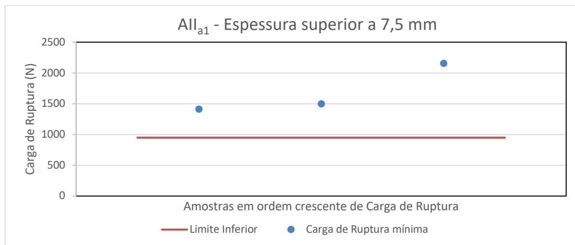
Figura 19: Valor mínimo de carga de ruptura dos produtos avaliados do grupo de absorção de água All_{a1} .
