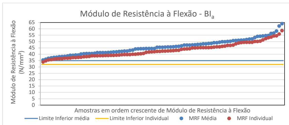
Figura 29: Valores médio e individual mínimo do módulo de resistência à flexão dos produtos do grupo de absorção de água BIa.
