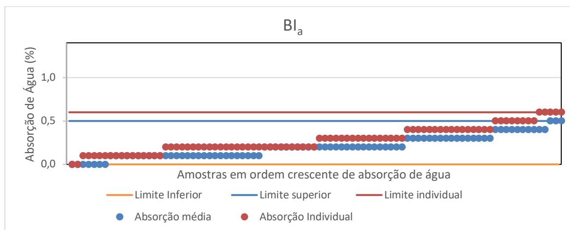
Figura 13: Valores médio e individual máximo de absorção de água para o produto do grupo de absorção de água Bl a .
