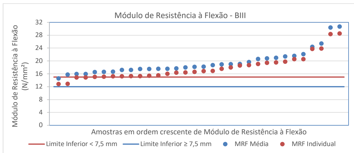
Figura 27: Valores médio e individual mínimo do módulo de resistência à flexão dos produtos do grupo de absorção de água BIII.
