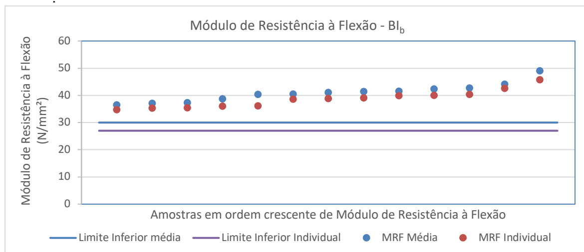
Figura 24: Valores médio e individual mínimo do módulo de resistência à flexão dos produtos do grupo de absorção de água BI b .
