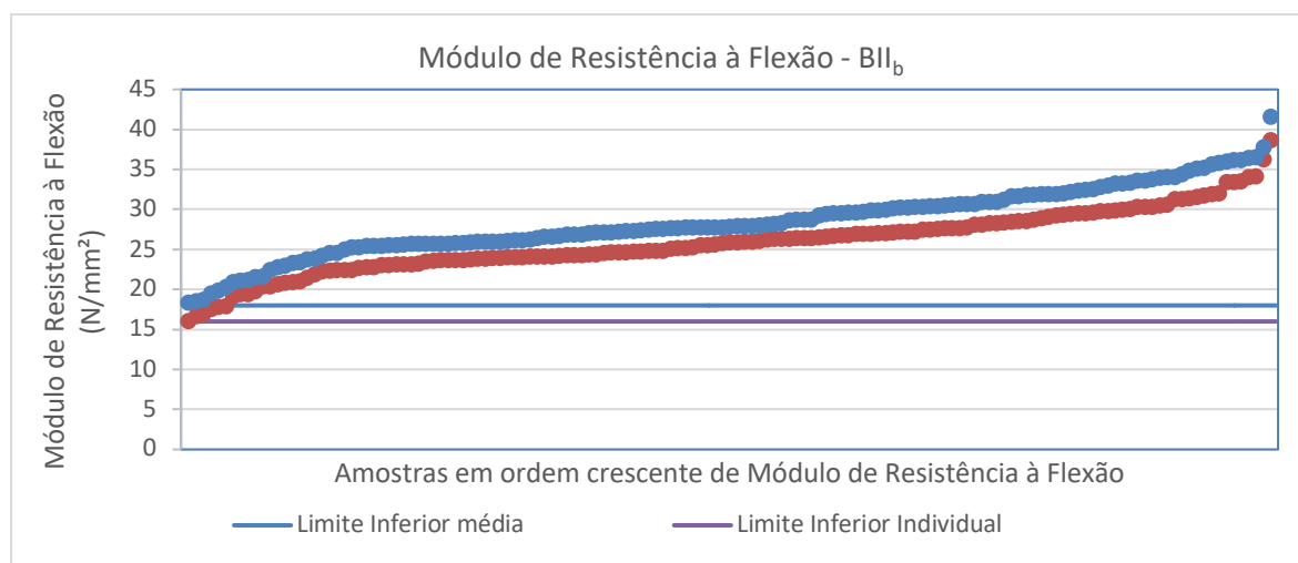
Figura 26: Valores médio e individual mínimo do módulo de resistência à flexão dos produtos do grupo de absorção de água BIIb.
