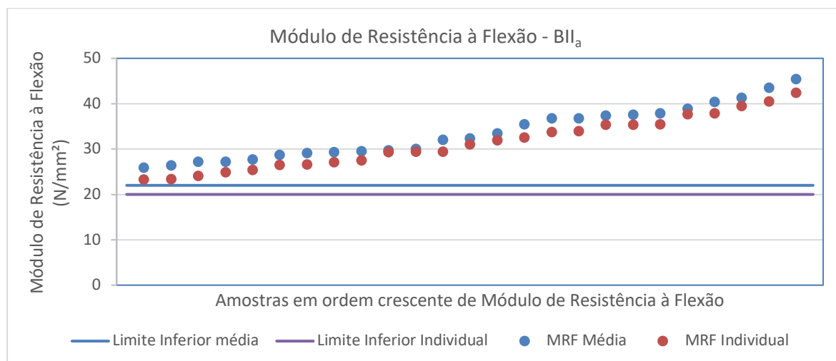
Figura 25: Valores médio e individual mínimo do módulo de resistência à flexão dos produtos do grupo de absorção de água BIIa.
