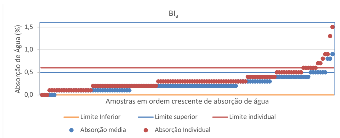
Figura 11: Valores médio e individual máximo de absorção de água para o produto do grupo de absorção de água BIa.
