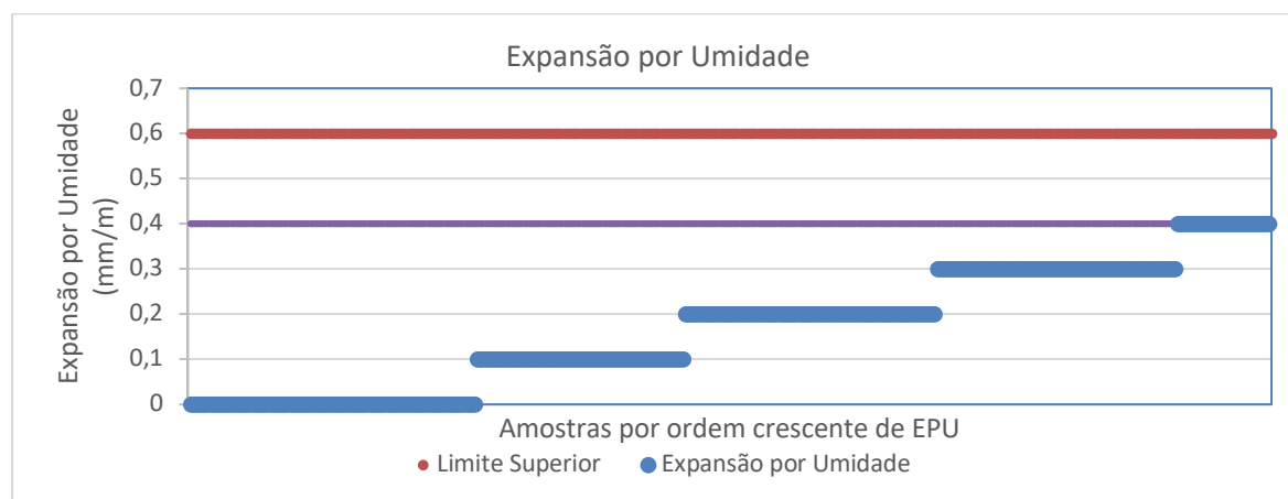
Figura 33: Resultados da determinação da expansão por umidade dos produtos.
