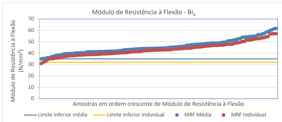
Figura 23: Valores médio e individual mínimo do módulo de resistência à flexão dos produtos do grupo de absorção de água BI a .
