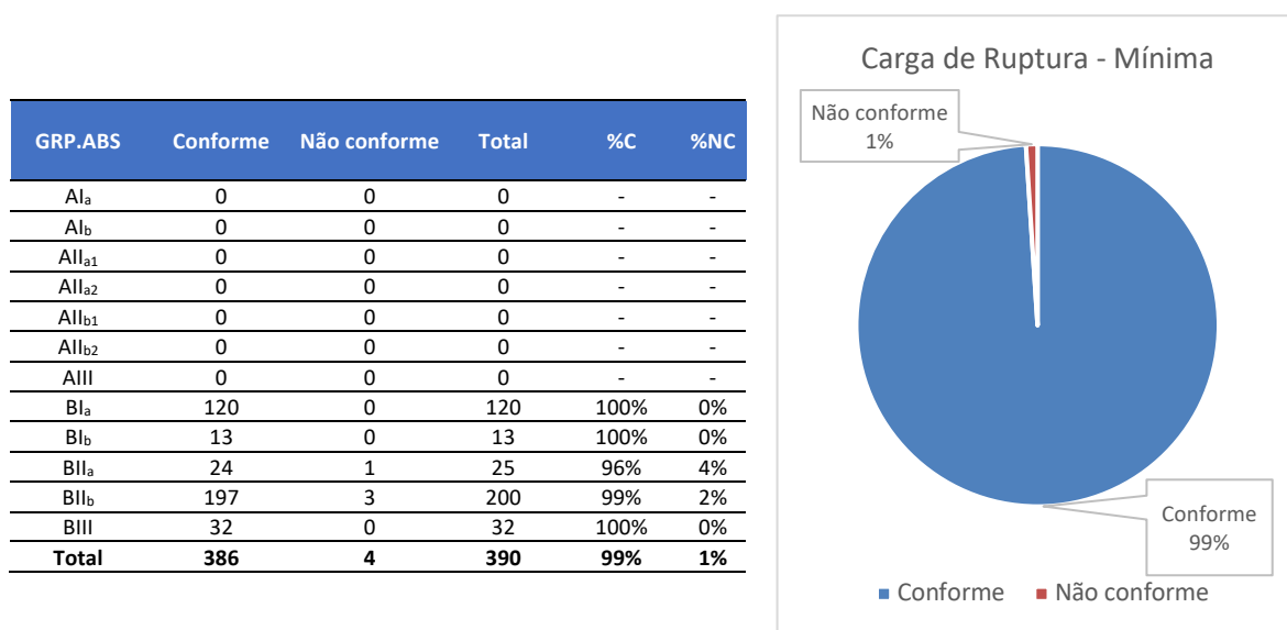
Figura 16: Conformidade de carga de ruptura de todos os grupos de absorção de água avaliados.
