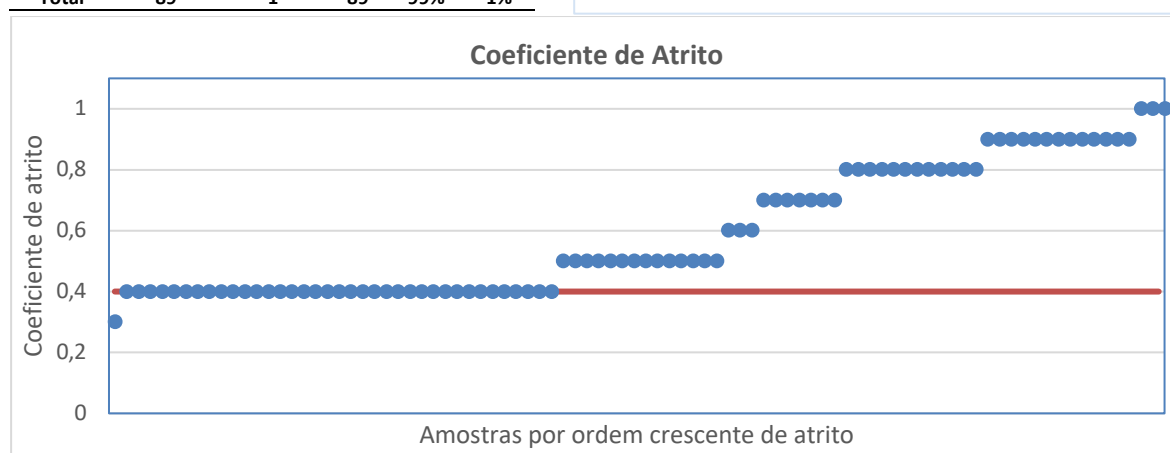
Figura 41: Resultados de determinação do coeficiente de atrito dos produtos avaliados.
