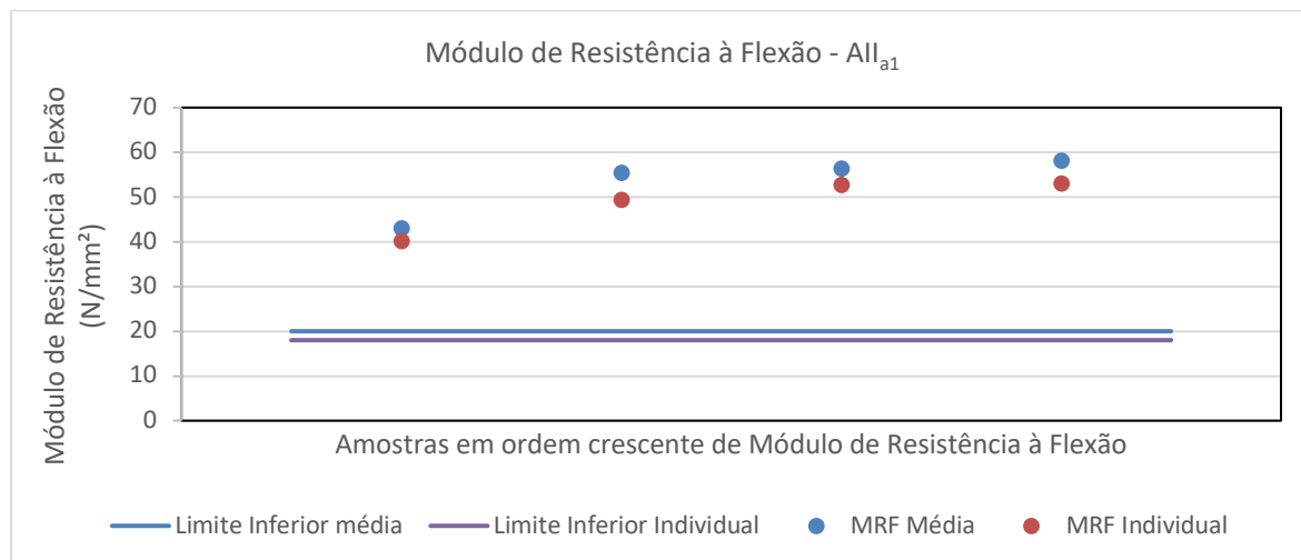
Figura 24: Valores médio e individual mínimo do módulo de resistência à flexão do produto do grupo de absorção de água All a1 .
