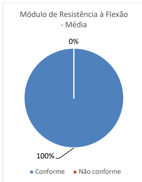
(a) Conformidade do valor médio de módulo de resistência a flexão em função dos grupos de absorção de água
