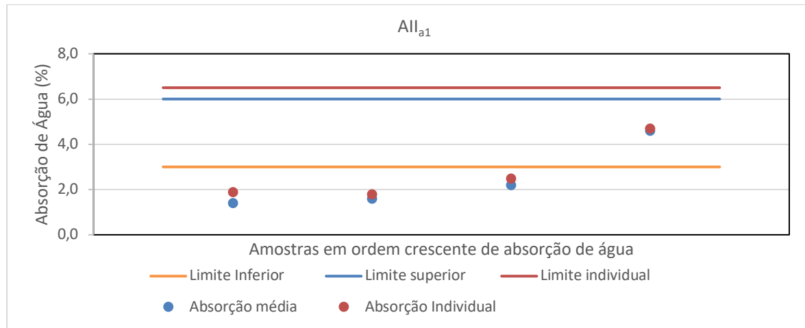
Figura 10: Valores médio e individual máximo de absorção de água para o produto do grupo de absorção de água All_{a1} .
