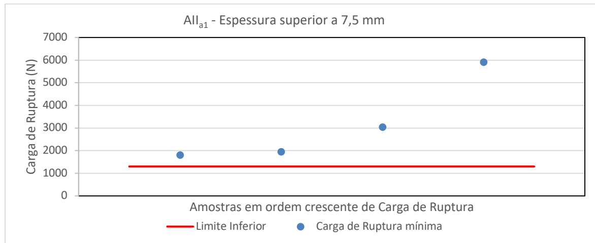
Figura 17: Valor mínimo de carga de ruptura dos produtos avaliados do grupo de absorção de água All_{a1} .
