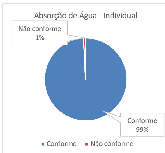
(b) Conformidade referente ao valor individual máximo de absorção de água de todos os produtos avaliados
