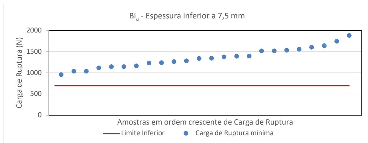
(a) Produtos com espessura inferior a 7,5 mm
